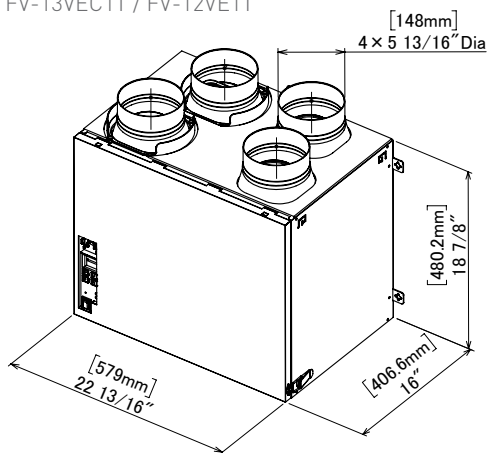
FV-16VEC1T / FV-15VE1T / FV-13VEC1T / FV-12VE1T
