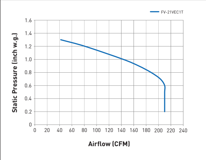
FV-21VEC1T Net Supply
