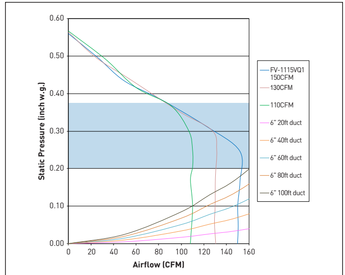
FV-1115VQ1 110-130-150 CFM 6" Duct
