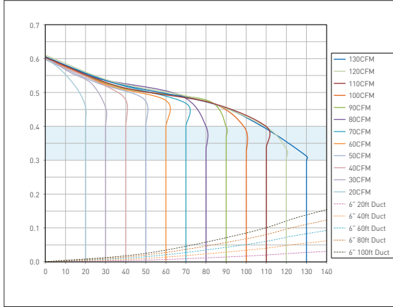
FV-13NLF51 / FV-13NLF5C1
