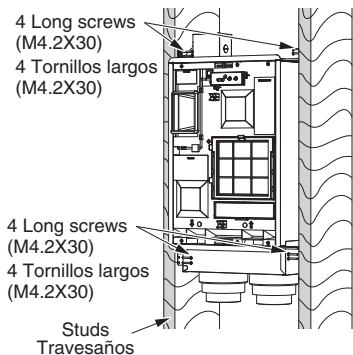
Suspension bracket Anclaje de suspensión
