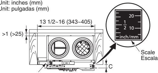
Suspension bracket Anclaje de suspensión
